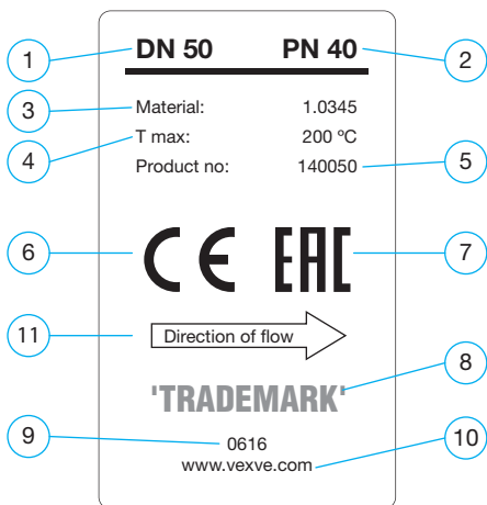
Рис. 1. Заводская табличка
